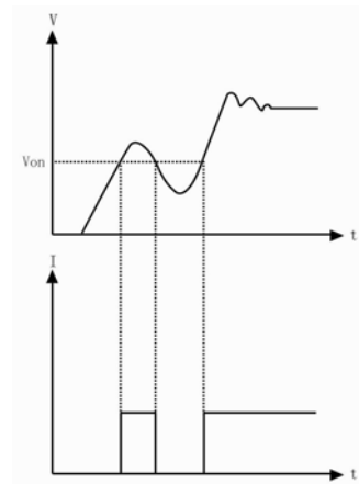
图 2-12 启动电压锁定(Von Latch)关闭
