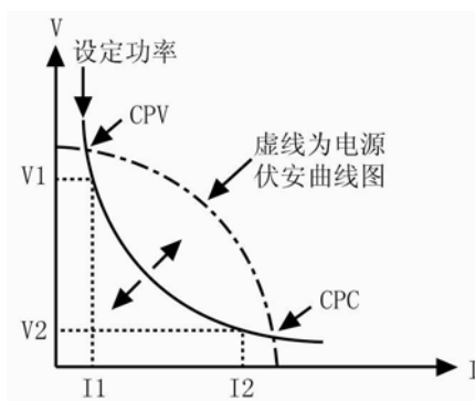
图 2-4 恒功率模式
