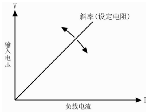
图 2-3 定电阻模式
