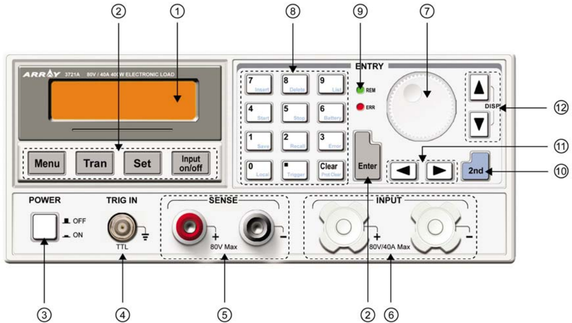
图 1-1 前面板图
