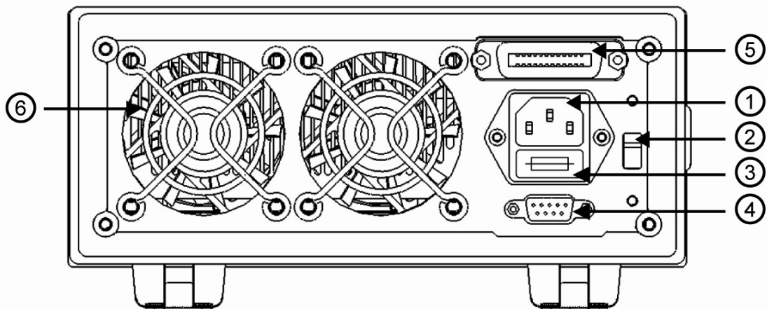
图 1-2 后面板图
