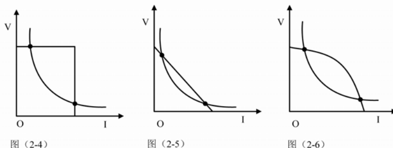
2-5 常见电源的伏安曲线
