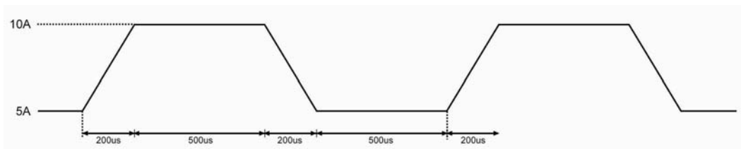
图 2-6 连续方式
