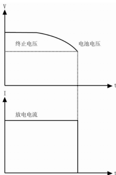
图 2-10 电池容量测试时电压、电流曲线
