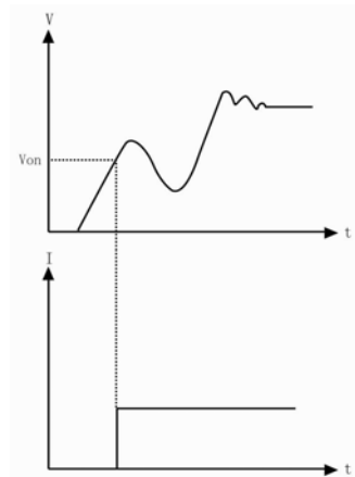
图 2-11 启动电压锁定(Von Latch)打开
